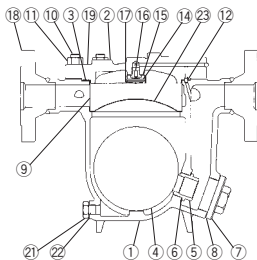
JH8R-X
